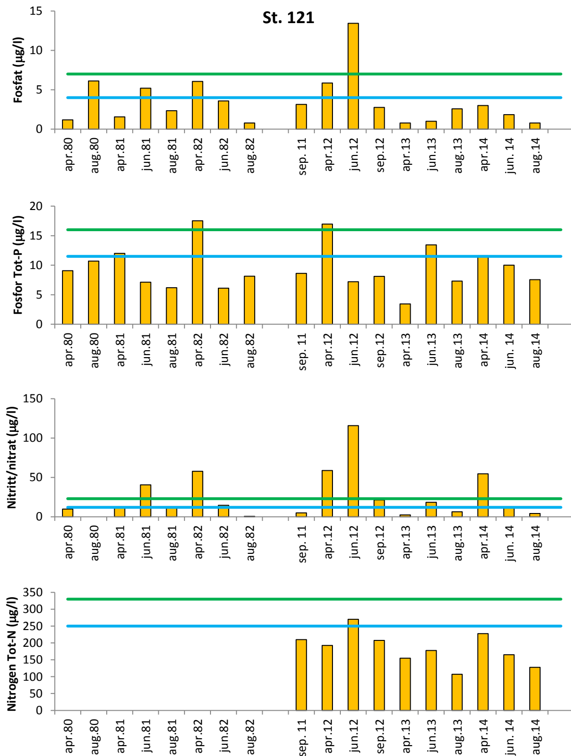
Figur 3.1.6 Gjennomsnittlig konsentrasjon av fosfat, nitrat/nitritt, total fosfor og total mengde nitrogen i prøver fra overflatelaget (0-10 m dyp) ved St. 121 i sommerhalvåret fra 2014 med historiske data. Miljødirektoratet grense for tilstandsklasser I og II for vinterhalvåret er markert med henholdsvis blå og grønn linje.
