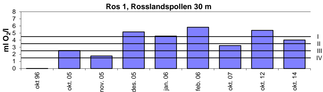
Figur 3.9.5 Oksygeninnholdet i bunnvannet på stasjon Ros 1 i Rosslandspollen. Miljødirektoratets tilstandsklasser for oksygenkonsentrasjon i bunnvann er indikert.
