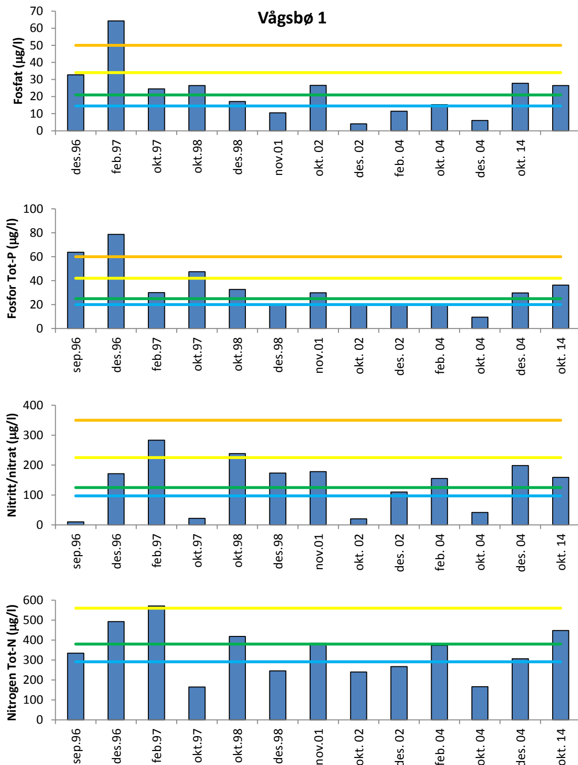
Figur 3.5.11 Gjennomsnittlig konsentrasjon av fosfat, nitrat/nitritt, total fosfor og total mengde nitrogen i prøver fra overflatelaget (0-10 m dyp) ved stasjon Vågsbø1 i vinterhalvåret tatt i perioden 2014 med historiske data. Miljødirektoratets øvre grense for tilstandsklasser I og II for vinterhalvåret er markert med henholdsvis blå og grønn linje.
