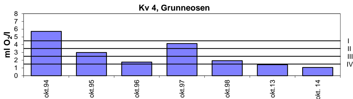
Figur 3.5.16 Oksygeninnholdet i bunnvannet på stasjon Kv4 i Grunneosen. Miljødirektoratets tilstandsklasser for oksygenkonsentrasjon i bunnvann er indikert.
