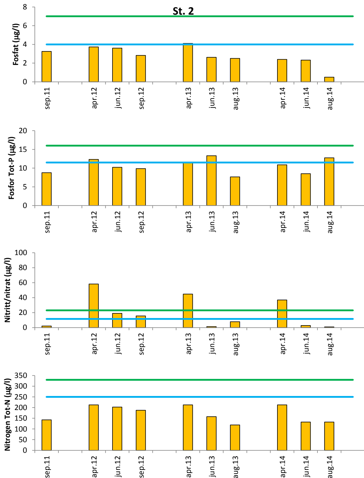
Figur 3.1.4 Gjennomsnittlig konsentrasjon av fosfat, nitrat/nitritt, total fosfor og total mengde nitrogen i prøver fra overflatelaget (0-10 m dyp) ved St. 2 i sommerhalvåret fra 2014 med historiske data. Miljødirektoratet grense for tilstandsklasser I og II for vinterhalvåret er markert med henholdsvis blå og grønn linje.
