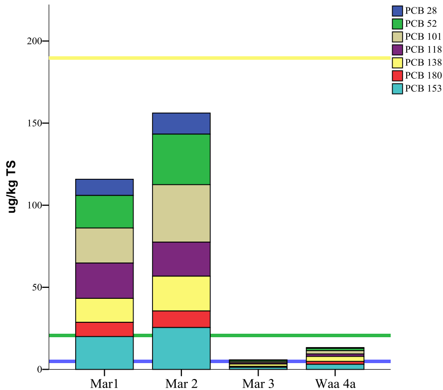
Figur 3.8.3 Innhold av PCB i sediment fra Marikoven i 2014, med de ulike PCB kongenerne som utgjør SumPCB7. De horisontale linjene representerer øvre grenseverdier for tilstandsklassene for sum PCB7. Fargekoder: Blå = tilstandsklasse I; grønn= tilstandsklasse II; gul = tilstandsklasse III(TA 2229/2207)
